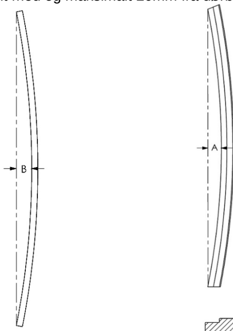
Krumning dørblade
