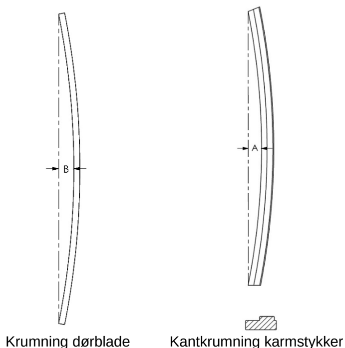
Figur 1. Principskitse for måling af krumninger
